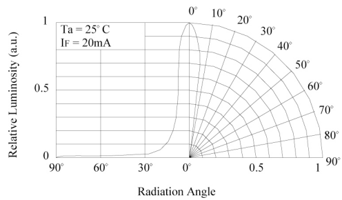
Directivity (Angle : 15°)
